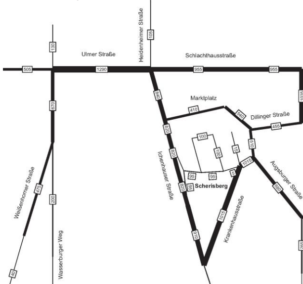
Verkehrsführung Variante 1 in Kfz/24 Stunden
