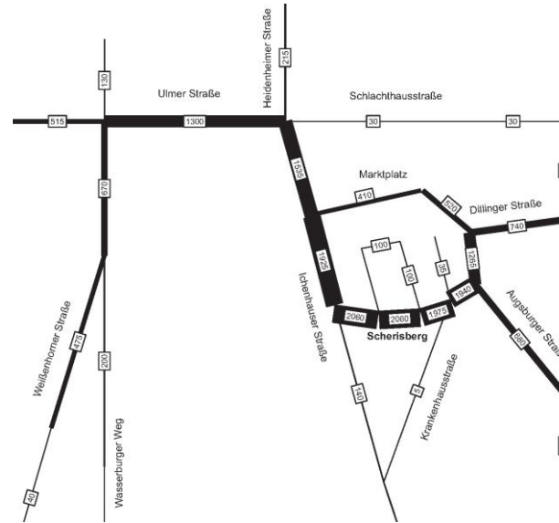
Verkehrsführung Bestand 2008 in Kfz/24 Stunden
